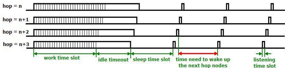
唤醒最坏情况示意图
