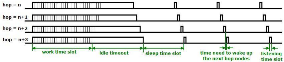
唤醒最理想情况示意图
